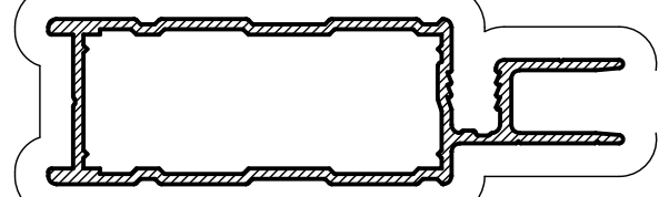
SD8 DOOR FRAME Mass. 0,629 Kg/m Anod. Per. 232 Paint Per. 197
